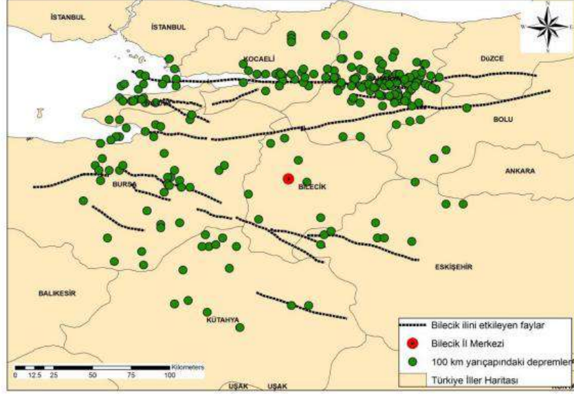
Bilecik İlini Etkileyen Faylar
